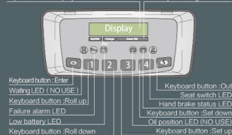
ZAPI Display
